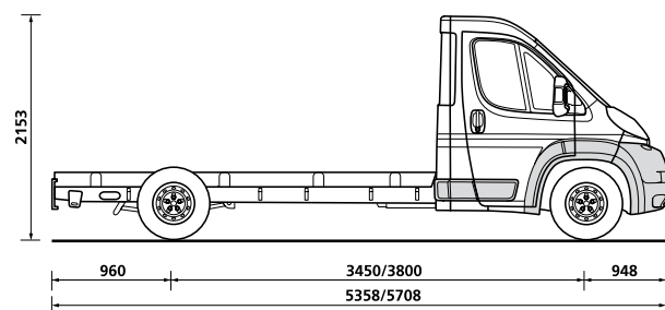
Châssis Cabine L2/L2S
