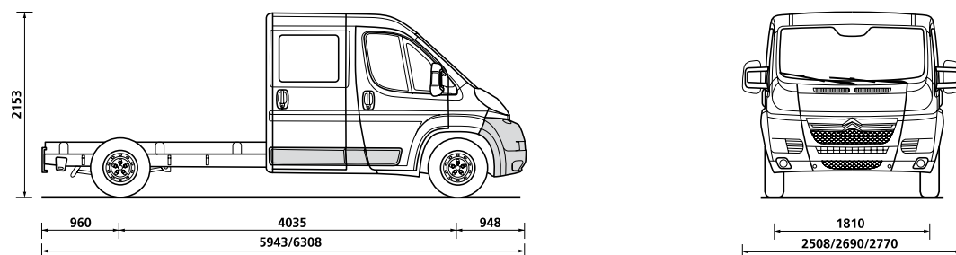
Châssis Double Cabine L3/L4
