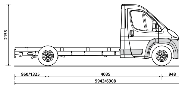
Châssis Cabine L3/L4
